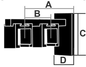
LA205DP SUPPORTO SQUARE DOPPIO SQUARE BRACKET-DOUBLE
