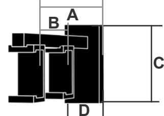
LA207DP SUPPORTO SHAPE DOPPIO SHAPE BRACKET-DOUBLE
