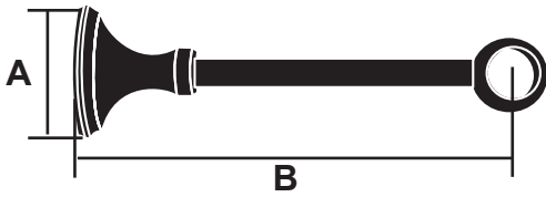
FA204 SATURNO APERTO SATURNO-OPENED
